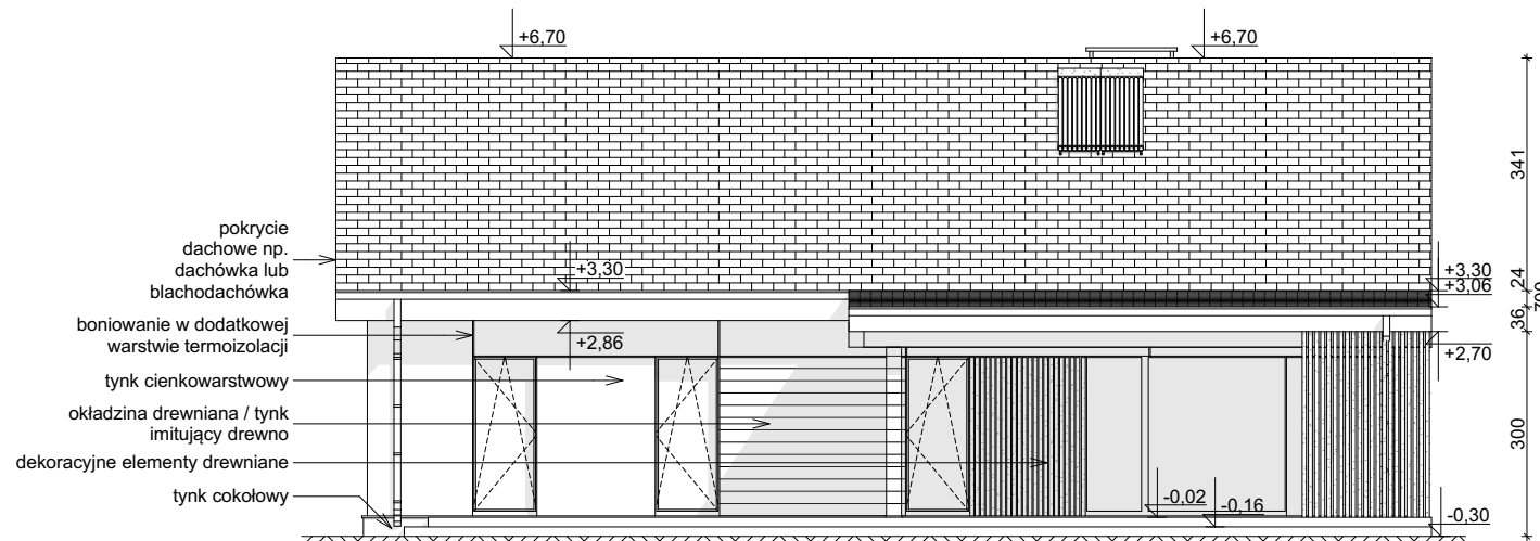
ELEWACJA OGRODOWA
