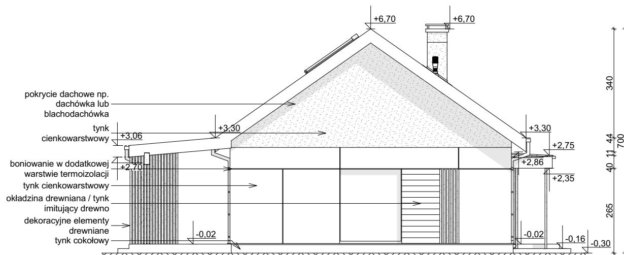
ELEWACJA BOCZNA
